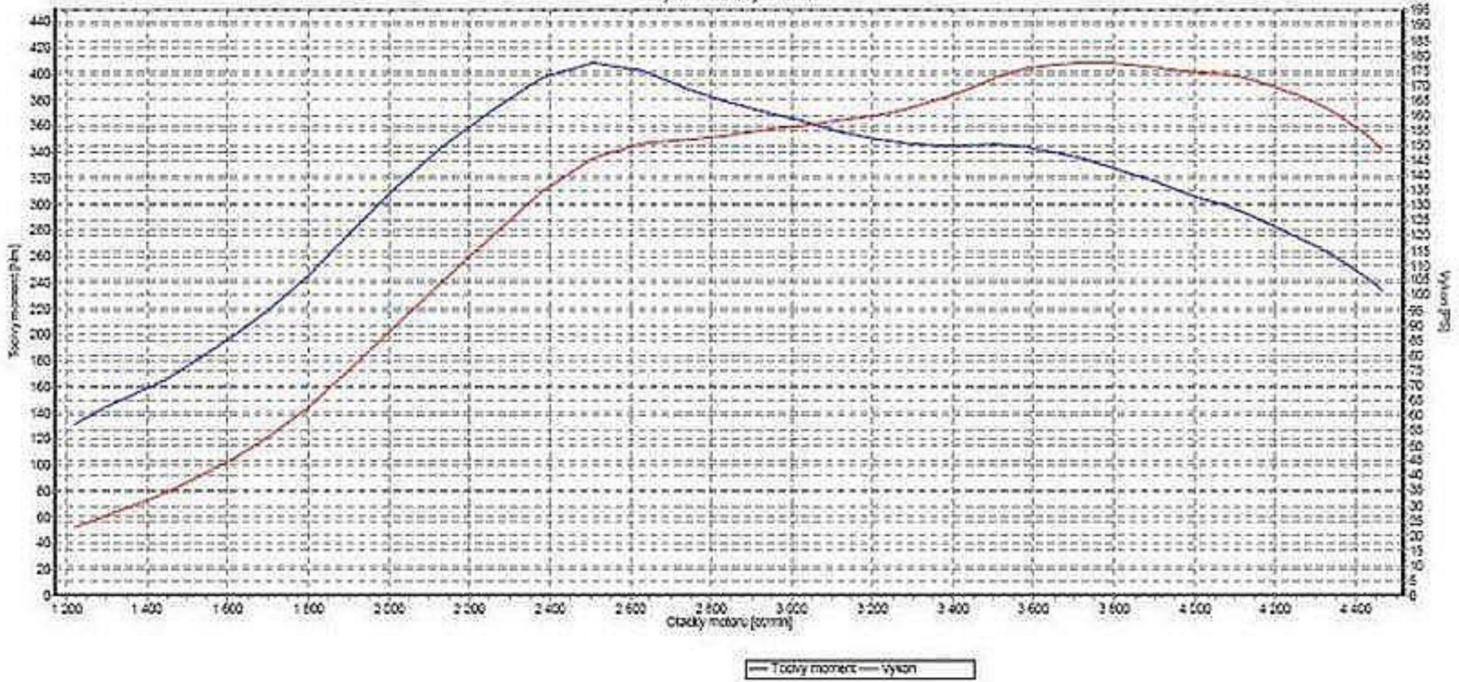
Tocivy moment a vykon motoru
